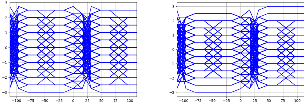
Figura 2.4.3: Diagrama de ojo S(3,2) truncado con \alpha = 0
