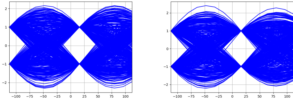
Figura 2.3.7: Diagrama de ojo S(8,7) rounded con \alpha = 0
