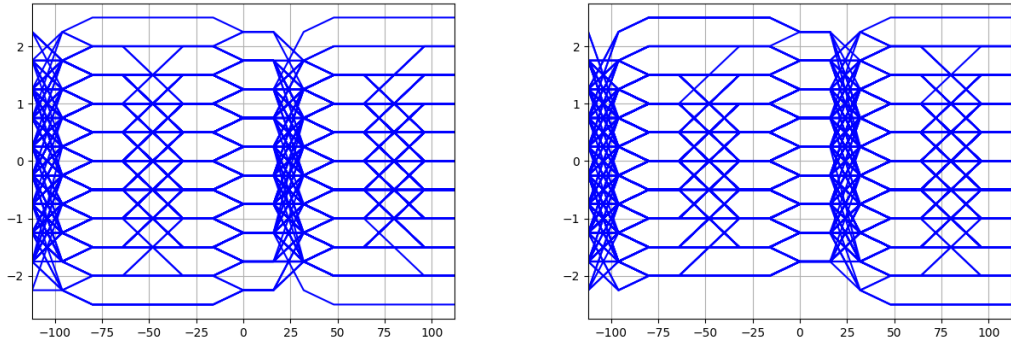
Figura 2.4.4: Diagrama de ojo S(3,2) truncado con \alpha = 0,5
