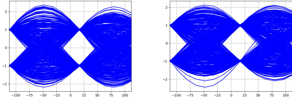
Figura 2.3.3: Diagrama de ojo S(8,7) truncado con \alpha = 0
