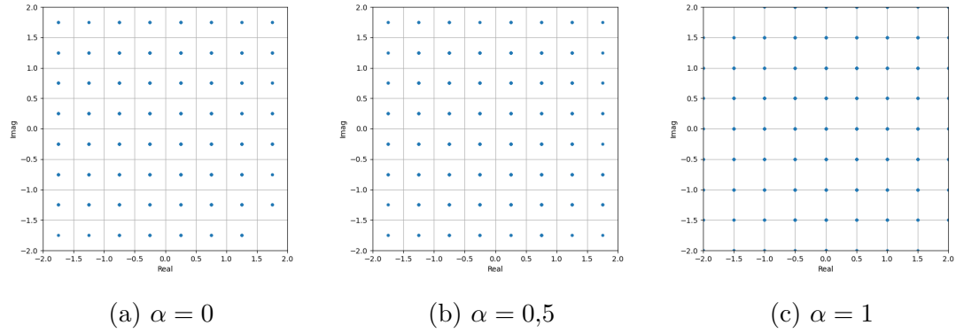
Figura 2.4.6: Constelaciones según \alpha para S(3,2) truncado
