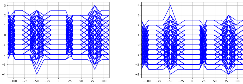
Figura 2.4.5: Diagrama de ojo S(3,2) truncado con \alpha = 1
